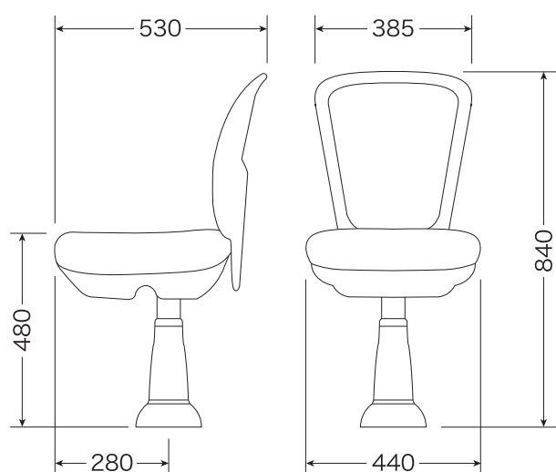
寸法図
