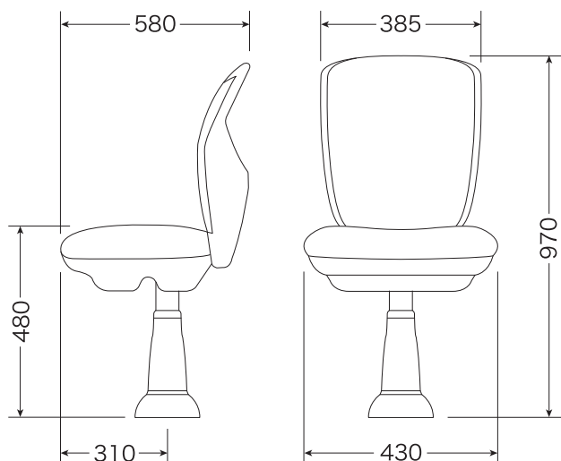
寸法図
