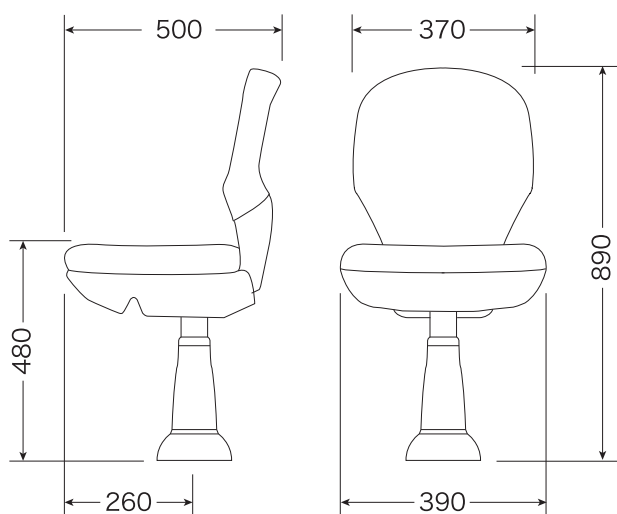
寸法図
