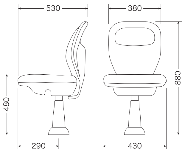
寸法図
